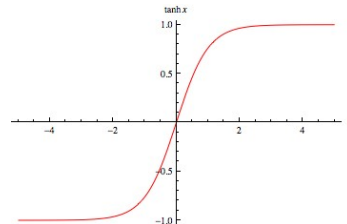
tanh
