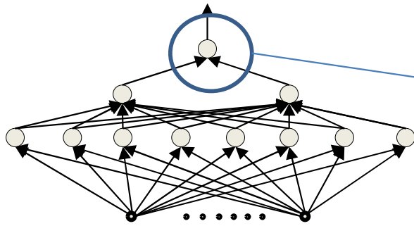
sigmoid
