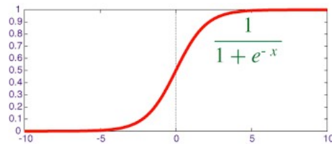
sigmoid
